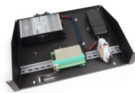
T8 reläenhet på ett 19" hyllplan med infästning och kablage för Sepura SRG/SCG22 (radioenhet ingår ej)
